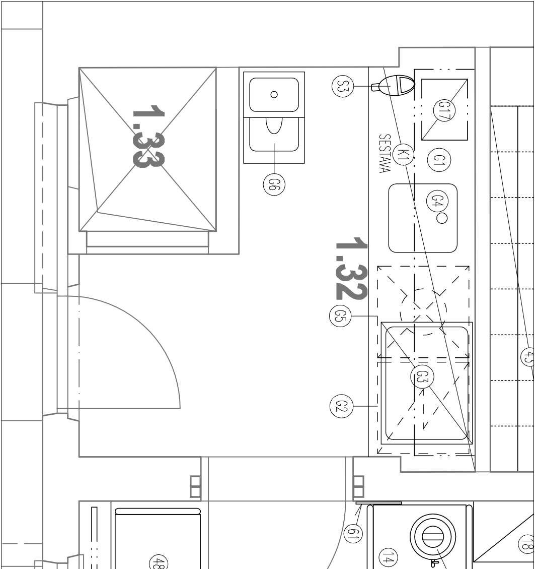
M.Č. 1.32 - PŘÍPRAVNA - VÝŘEZ
